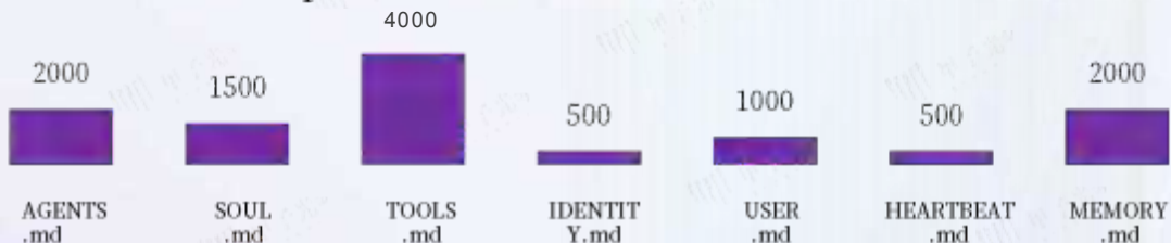
图3: OpenClaw每次对话携带文件的默认Tokens消耗数
